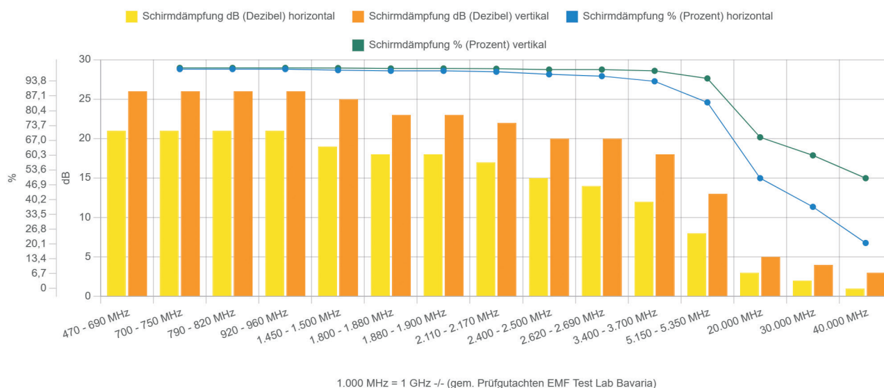
Schirmdämpfung - Antiwave OC weiß - stretched - 470 MHz bis 40.000 MHz (40 GHz)
